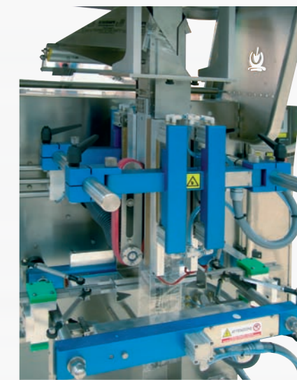
Dispositivo per buste a quattro saldature Four side seal device
